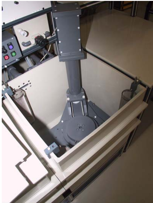
Innenansicht der 1. Beschichtungsstation mit Rotationseinheit horizontal
